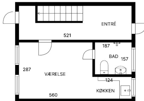
STUEPLAN
